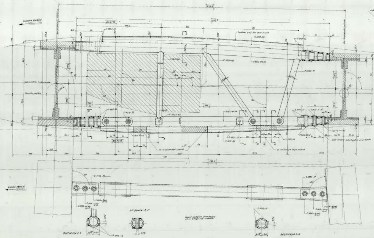
SECȚIUNEA F-F
