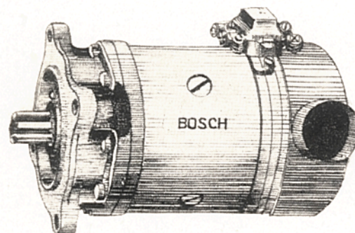
GENERATRICE 24V 600 BOSCH
